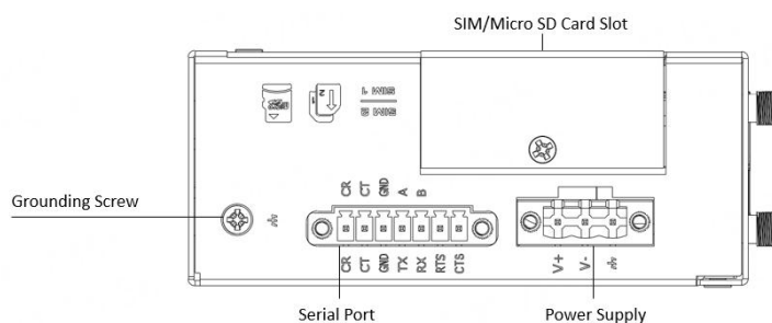
顶视图
