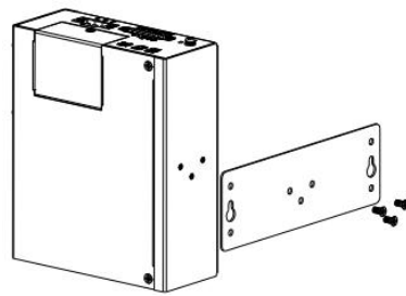
壁挂式安装
